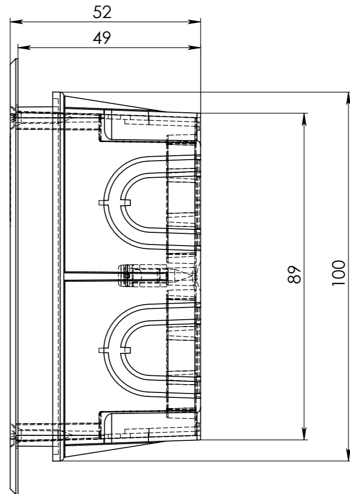
СЕЧЕНИЕ В-В МАСШТАБ 1 : 1
